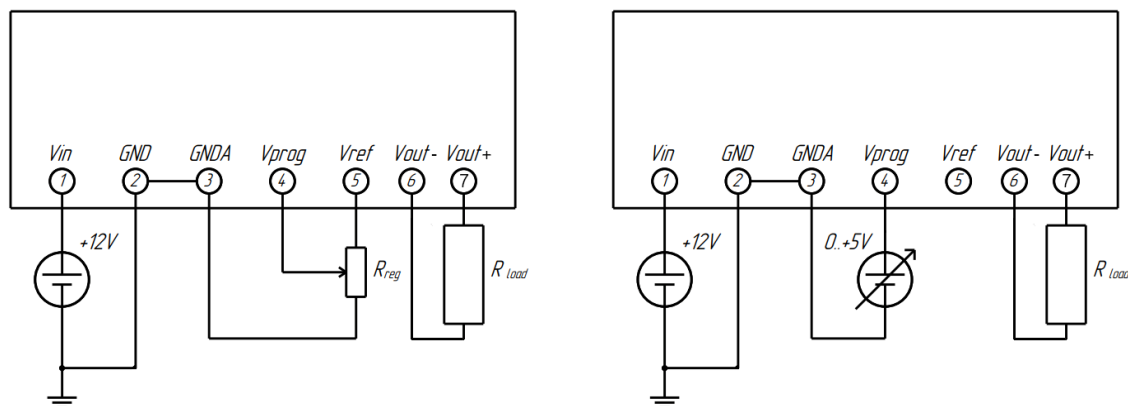
Рис. 2 – Схема подключения
